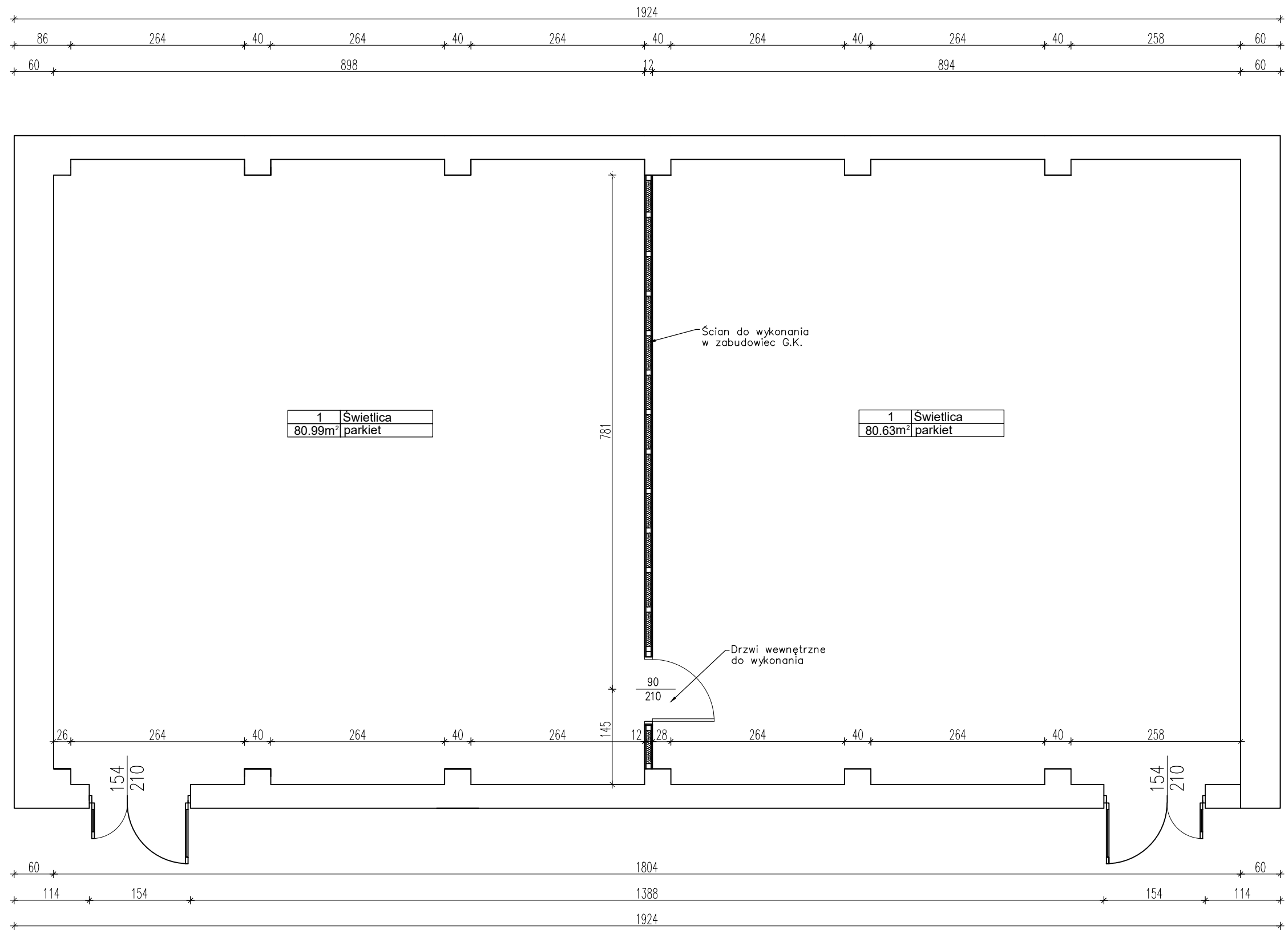
Rzut parteru-projektowany przekrój na rzędnej + 1,00
