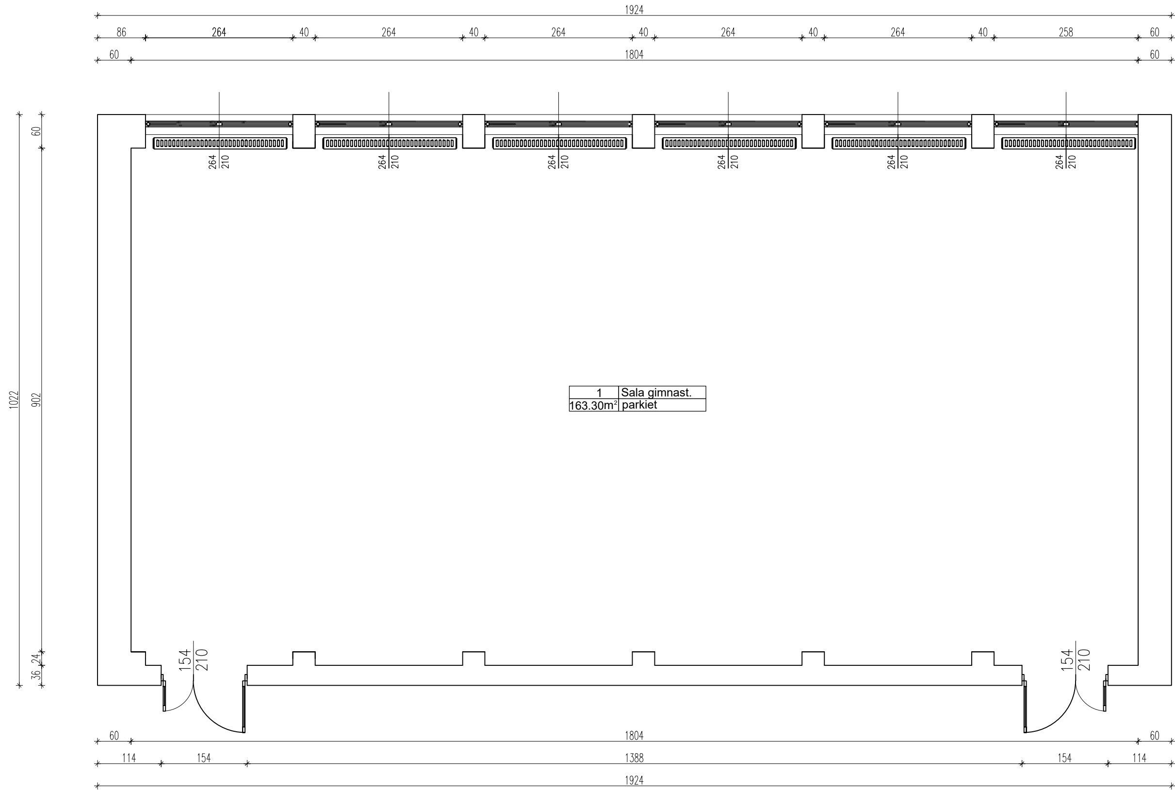
Rzut parteru-inwentaryzacja
